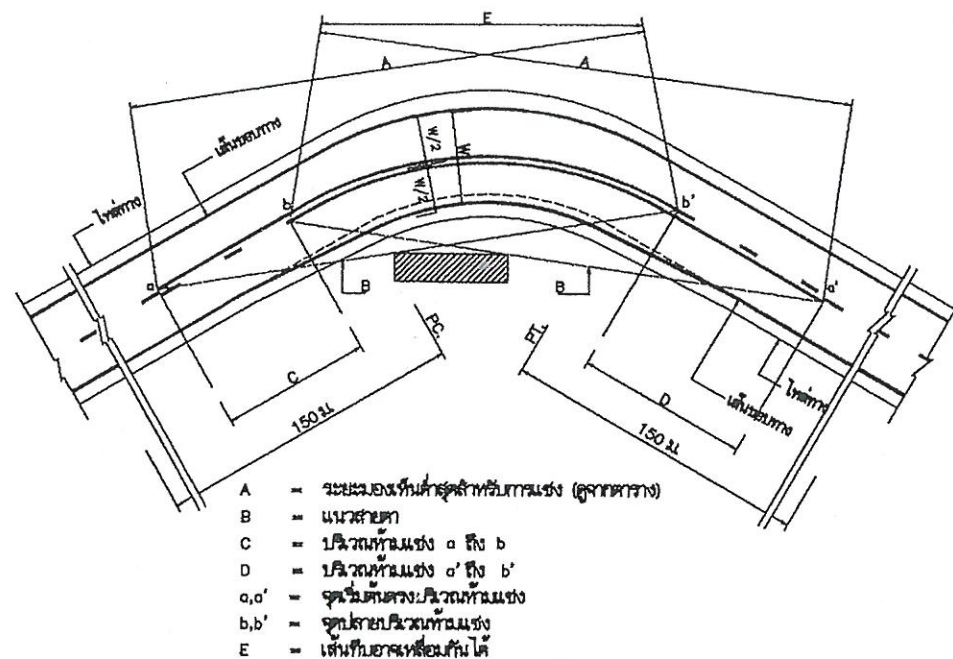
การเส้นจราจรบริเวณโค้งราบ
