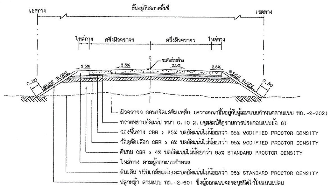
รูปตัดตามขวางแสดงดินตัดและดินถม
