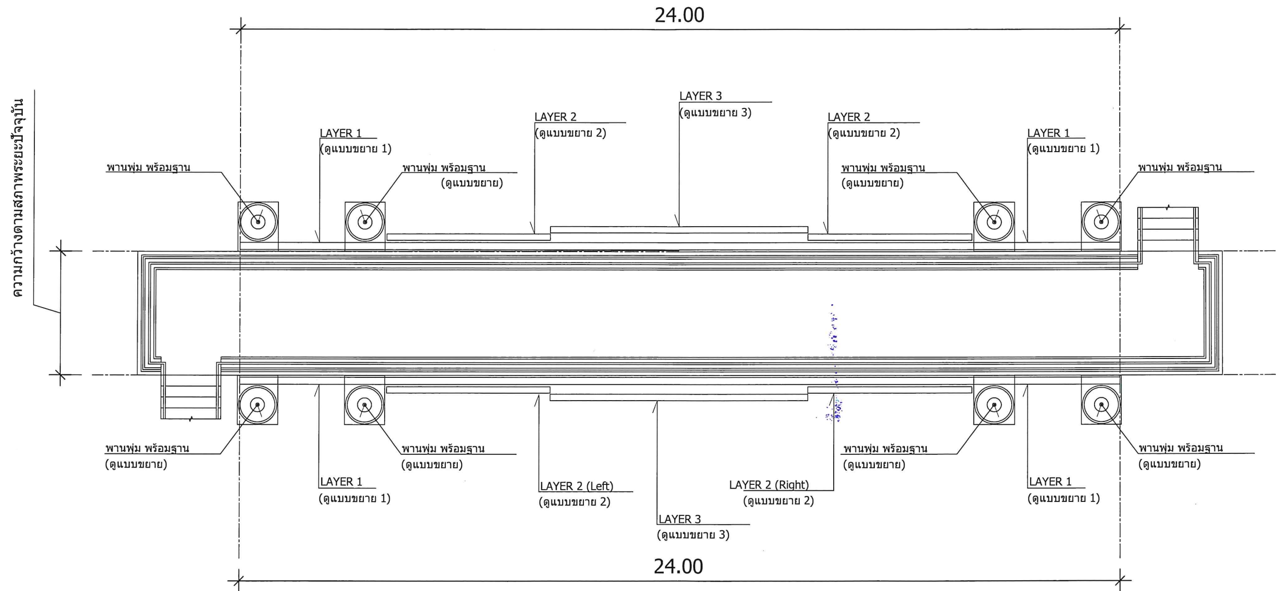
แปลน ติดตั้งชั้นประตึบนบนสะพานลอยคนข้าม ยาว 24 เมตร มาตรฐาน 1:100
