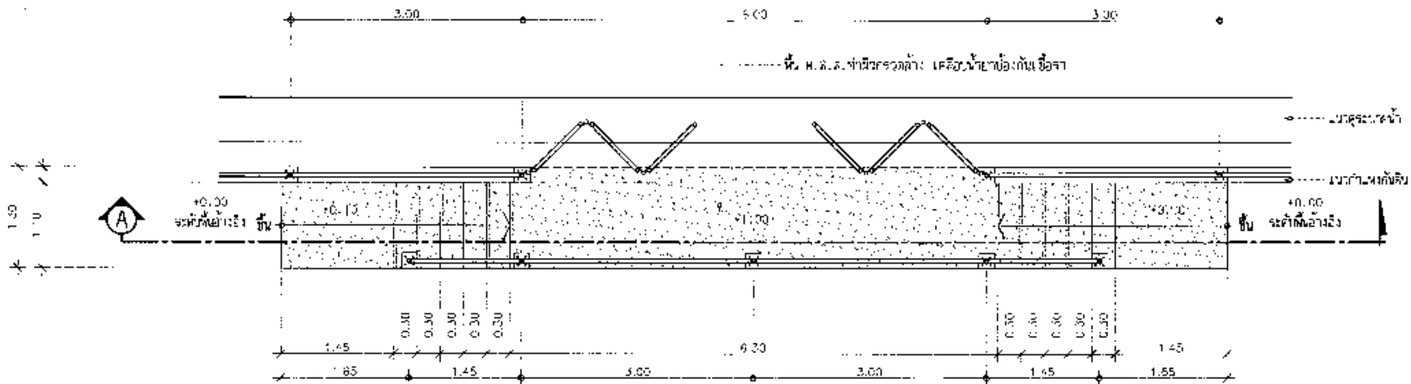
แบบขยายทางเข้าลำนามตำแหน่งที่ 1
