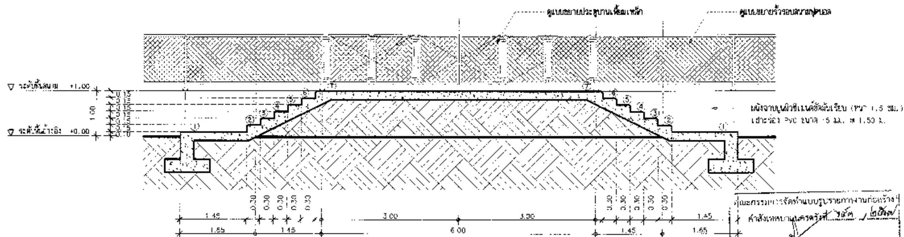
รูปตัด A ทางเข้าลำนามตำแหน่งที่ 1
