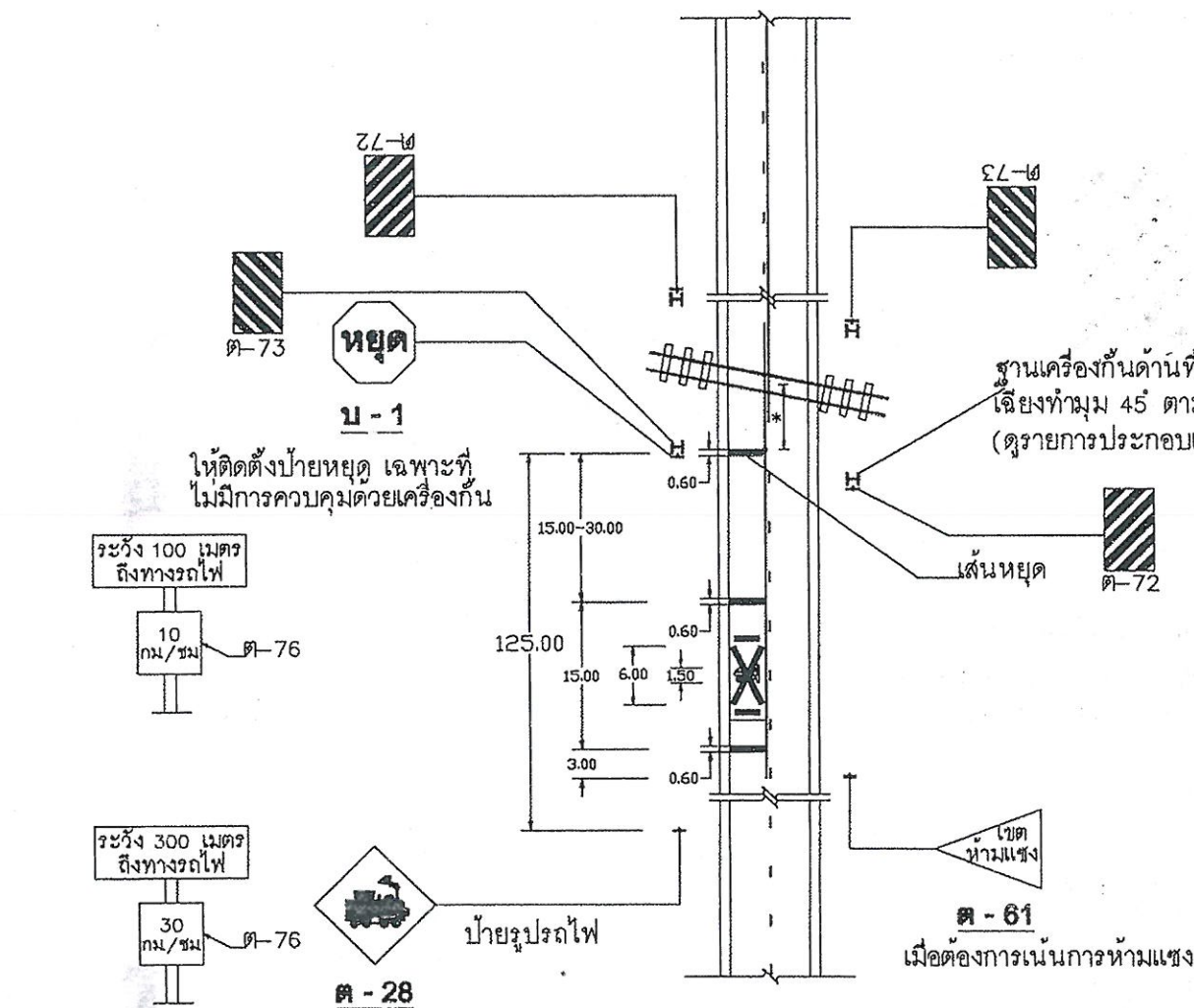
มาตรฐานการตีเส้นบริเวณทางรถไฟตัดผ่าน
