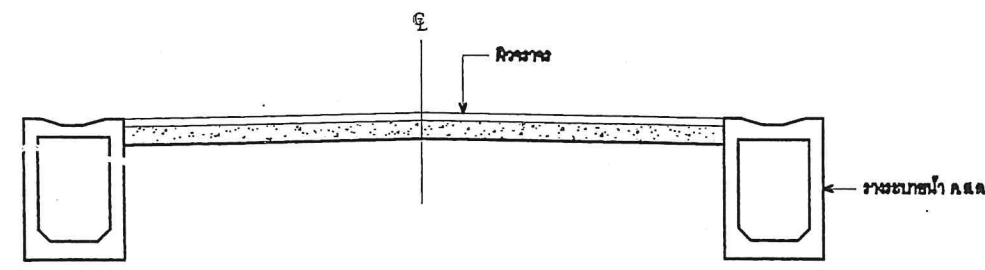
รูปตัดแสดงระดับวางระบายน้ำโดยประมาณ
