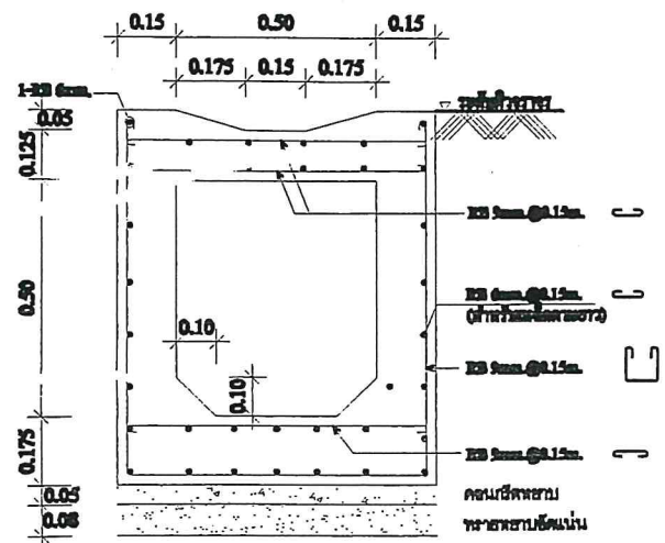
รูปตัด ๑-๑ พื้นรางดิน 1:20
