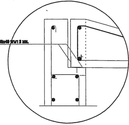
แบบขยาย 1 1:10
