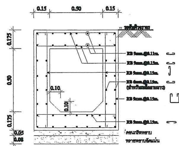
รูปตัดราง ก.ส.ถ.พื้นเรียบ 1:20
