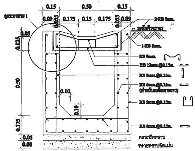
รูปตัด ๒-๒ ผ่ารางดิน 1:20
